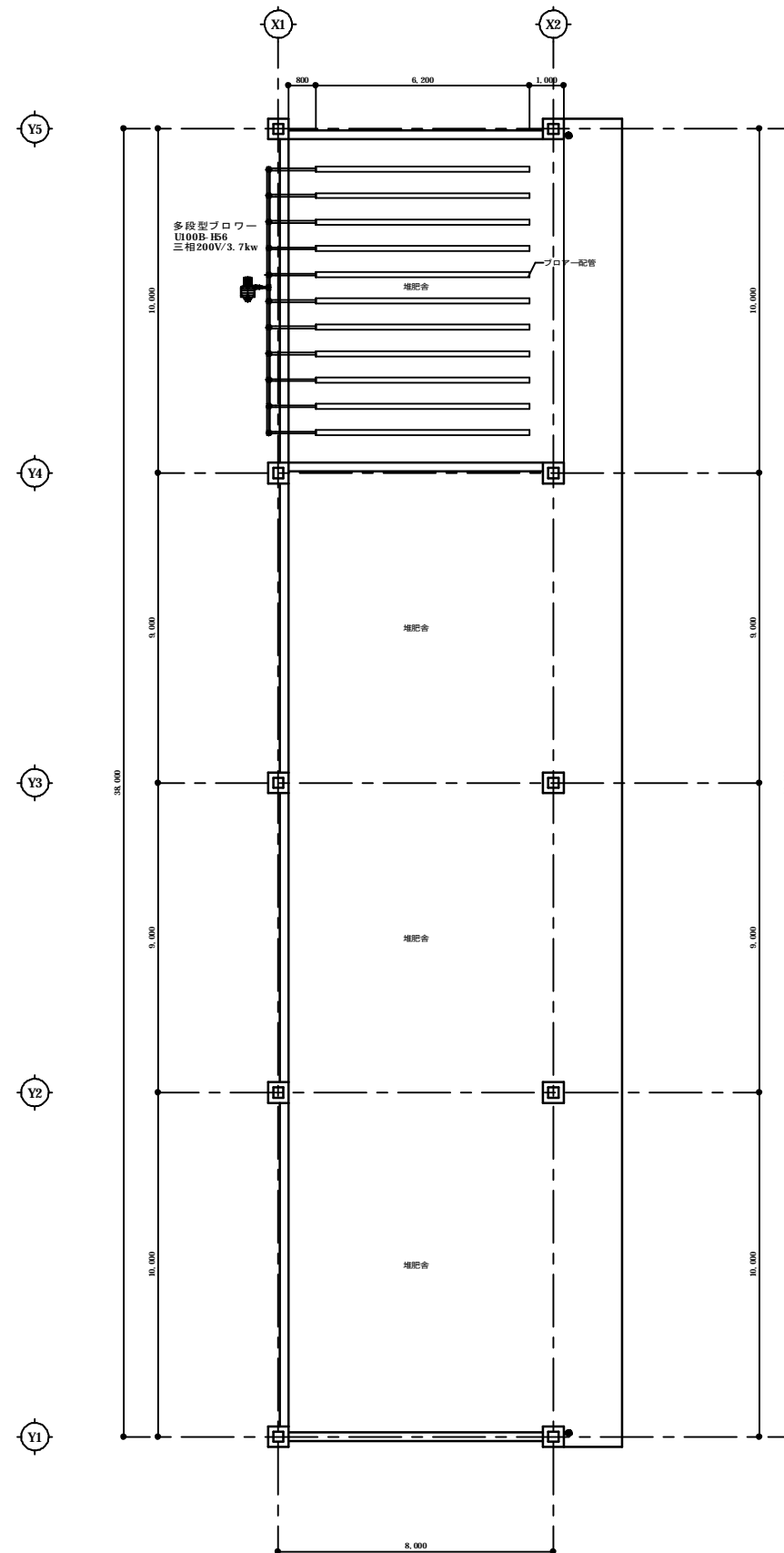
平面図 S=1/100
