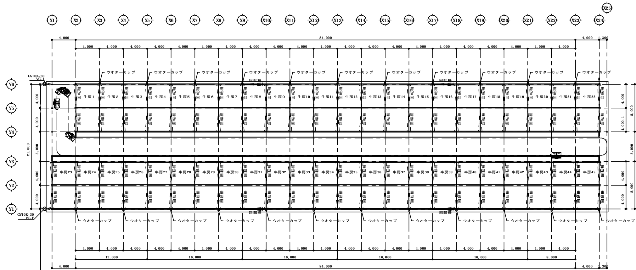
平面図 S=200
