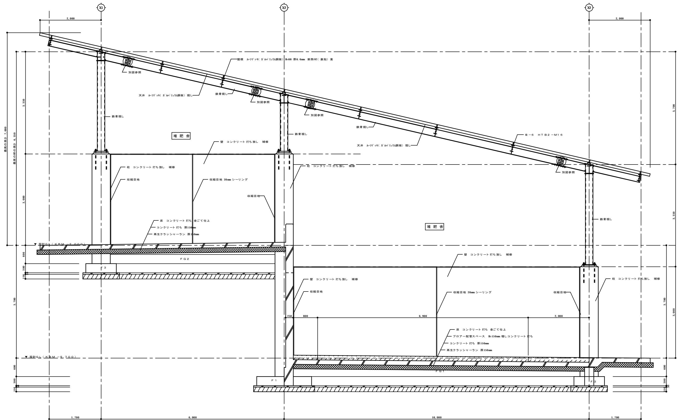
矩計図 S=1/30
