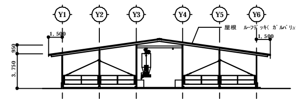
北側立面図 S=1/200
