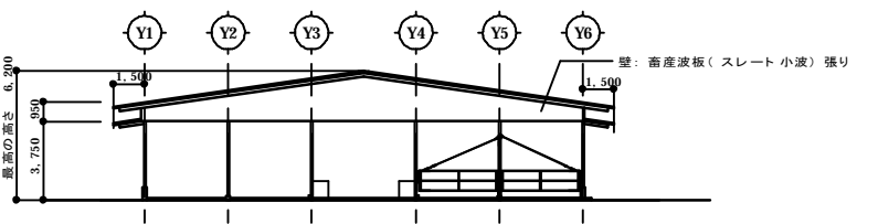
南側立面図 S=1/200
