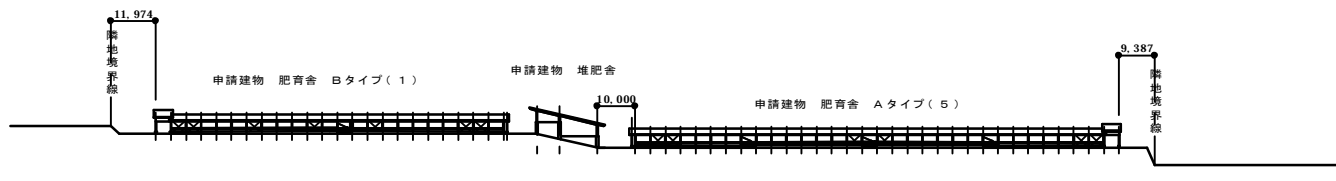
X-X断面図 S=1/1000
