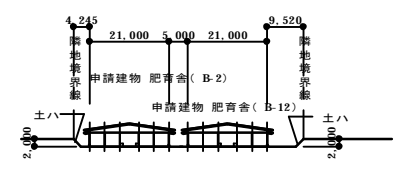
Y-Y断面図 S=1/1000
