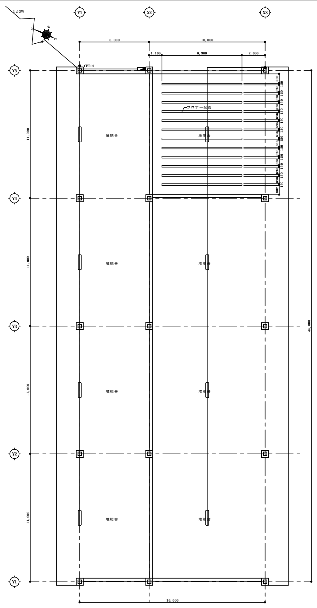
平面図 S=1/100
