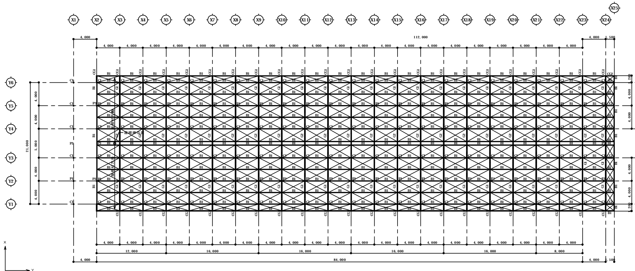
小屋伏図 S=200
